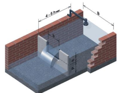
Obdélníkový přeliv
